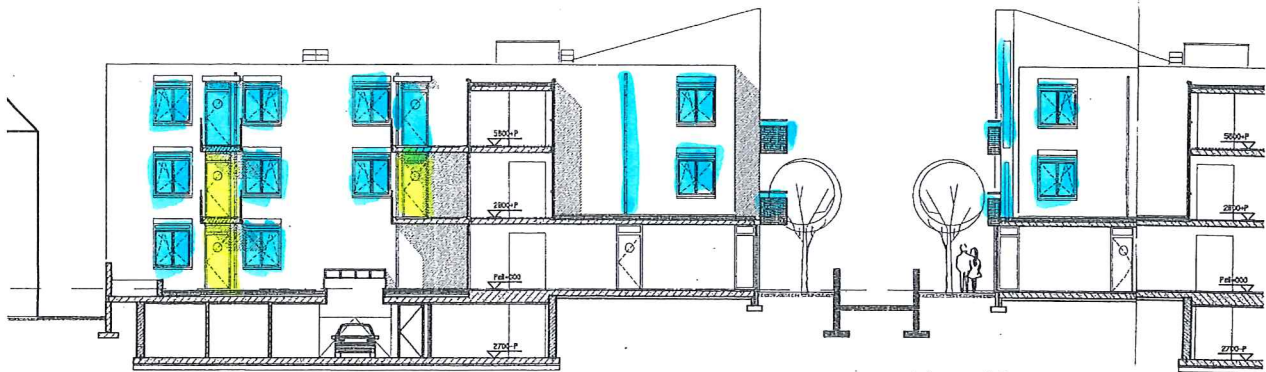
Achtergevel Grotestraat
