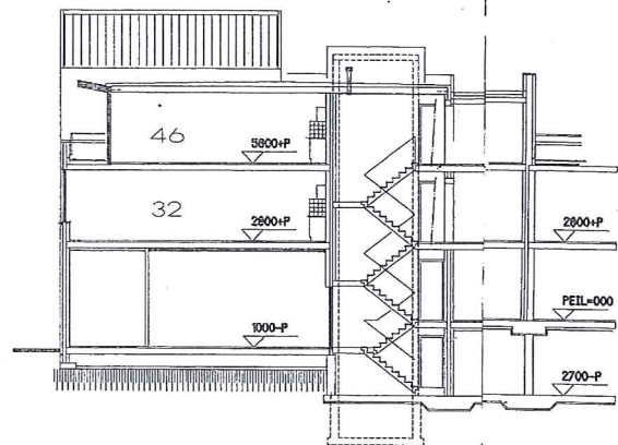
Doorsnede B-B
